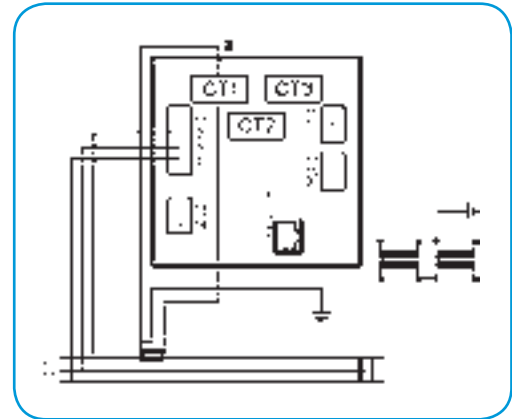
3b – трехфазное, трехпроводниковое, симметричная нагрузка
