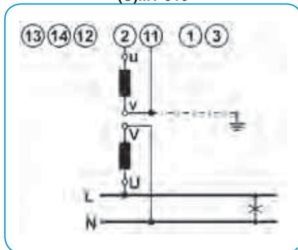
1b – однофазное
