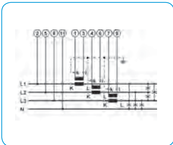
4и – трехфазное, четырехпроводниковое, несимметричная нагрузка
