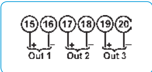
Преобразователь MI 400 может иметь до трех аналоговых выходов.
