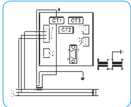
3b – трехфазное, трехпроводниковое, симметричная нагрузка
