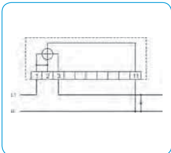
1b – однофазное, симметричная
