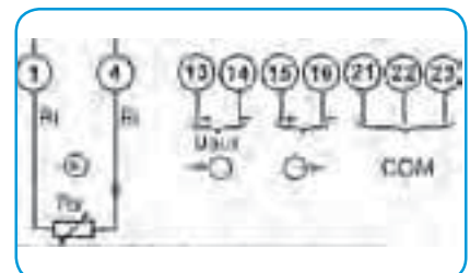
MI 450, 2-четырёхпроводный
