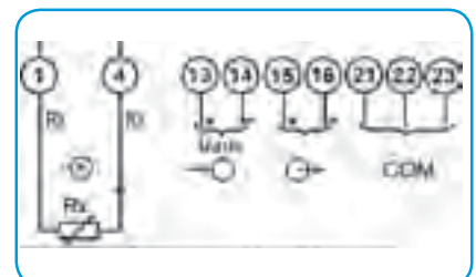
MI 452, 2-четырёхпроводный
