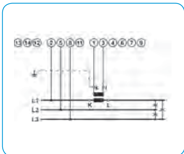
3b – трехфазное, трехпроводниковое, симметричная нагрузка
