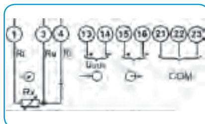
MI 452, 3-четырёхпроводный
