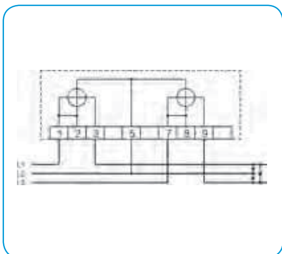
3и – трехфазное, трехпроводниковое, несимметричная нагрузка
