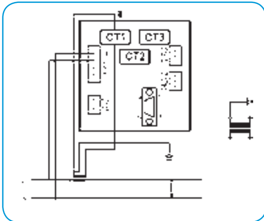
1b – однофазное, симметричная нагрузка
