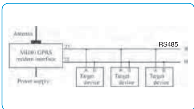
Подключение модем-адаптера
