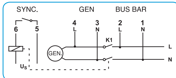
Соединительная схема фазного подключения
