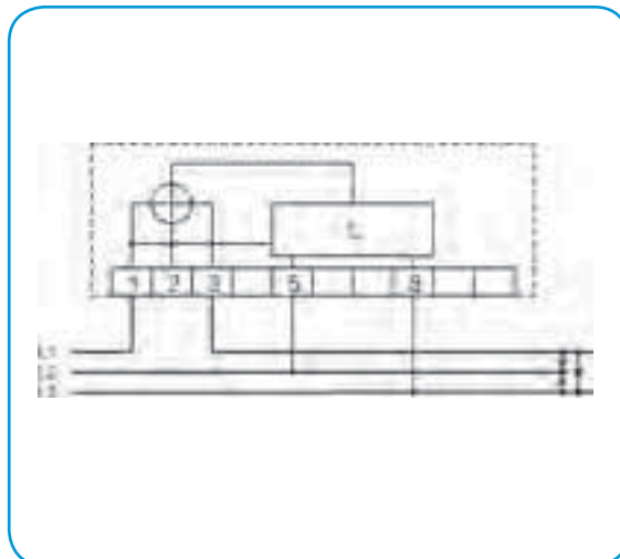
3b – трехфазное, трехпроводниковое, симметричная нагрузка
