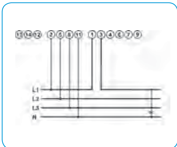
4b – трехфазное, четырехпроводниковое, симметричная нагрузка
