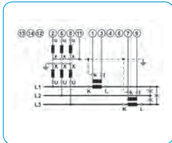
3u – трехфазное, трехпроводниковое, несимметричная нагрузка
