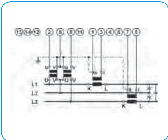
3u – трехфазное, трехпроводниковое, несимметричная нагрузка
