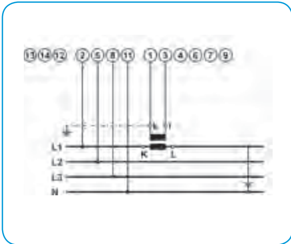
4b – трехфазное, четырехпроводниковое, симметричная нагрузка
