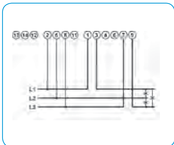
3и – трехфазное, трехпроводниковое, несимметричная нагрузка
