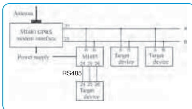
Подключение измерительного прибора через адаптер MI 485
