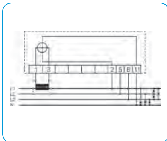
4b – трехфазное, четырёхпроводниковое, несимметричная
