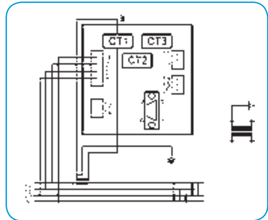
4b – трехфазное, четырехпроводниковое, симметричная нагрузка
