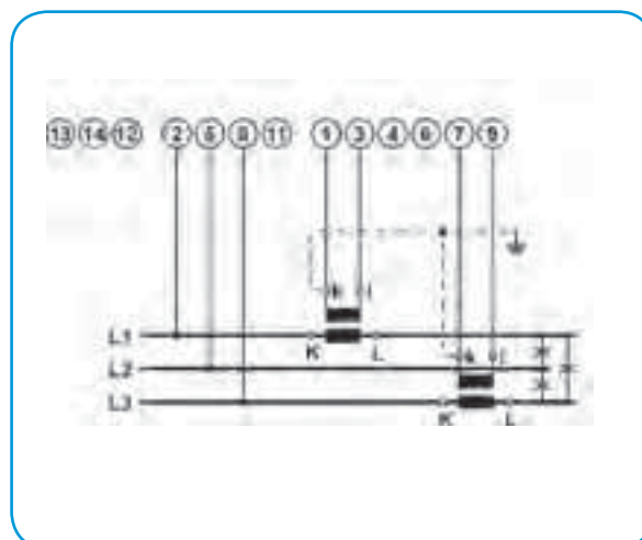
3и – трехфазное, трехпроводниковое, несимметричная нагрузка
