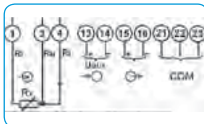
MI 450, 3-четырёхпроводный
