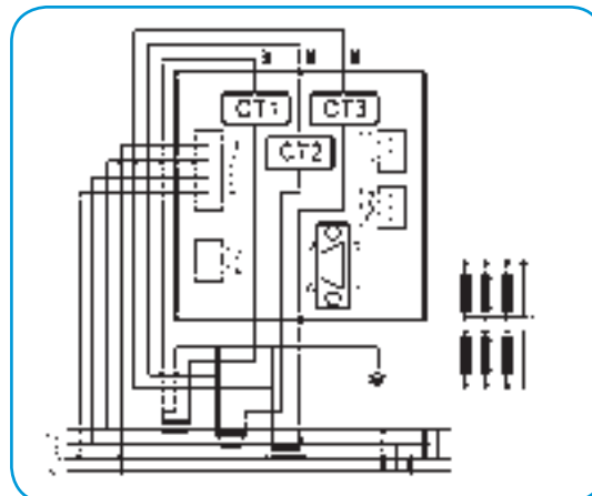
4и – трехфазное, четырехпроводниковое, несимметричная нагрузка
