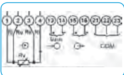
MI 452, 4-четырёхпроводный
