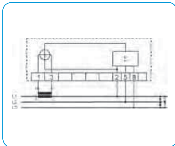
3b – трехфазное, трехпроводниковое, симметричная нагрузка
