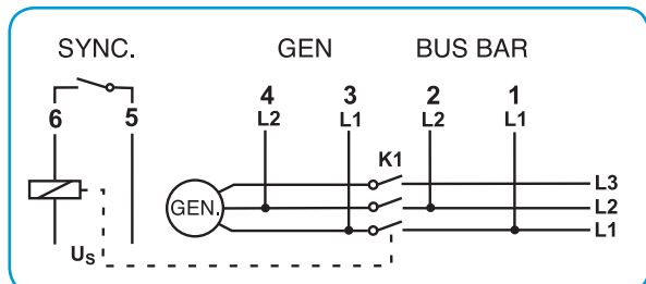
Соединительная схема межфазного подключения
