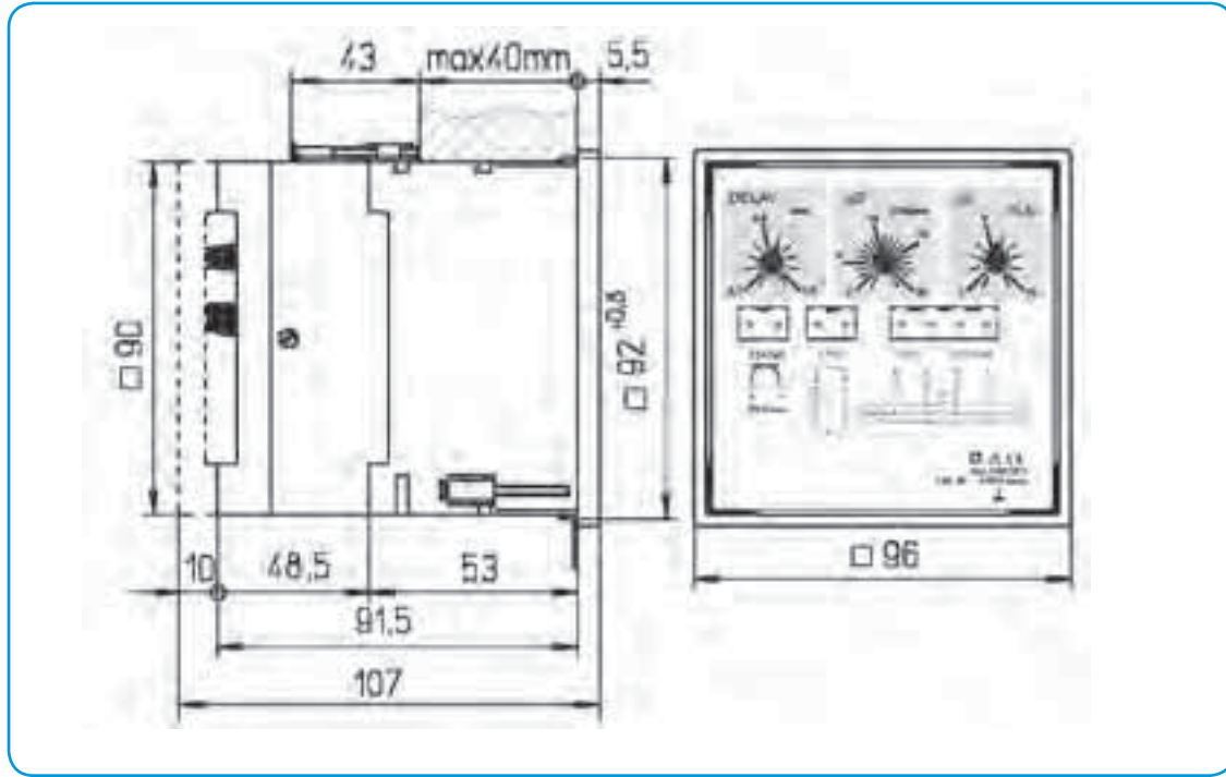
Синхрооскоп
