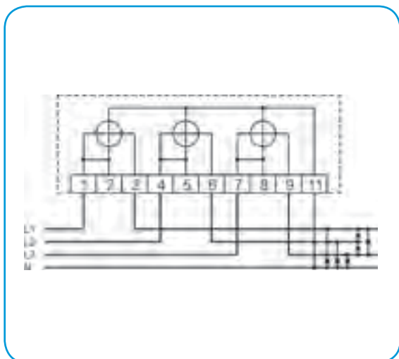
4и – трехфазное, четырехпроводниковое, несимметричная нагрузка
