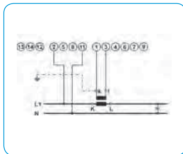
1b – однофазное
