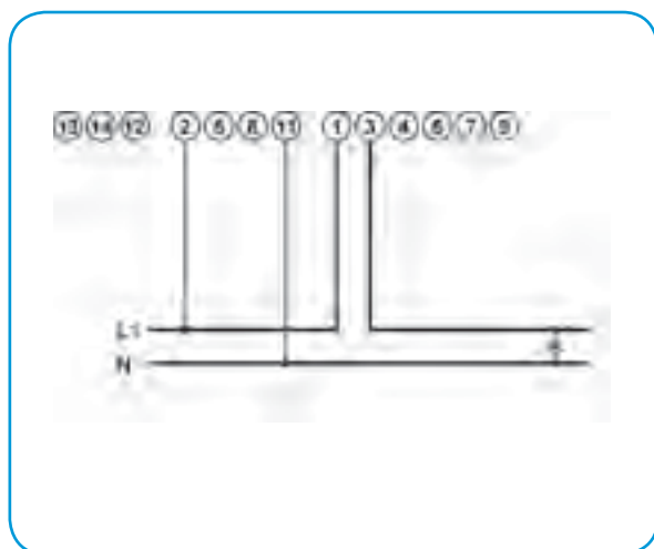
1b – однофазное
