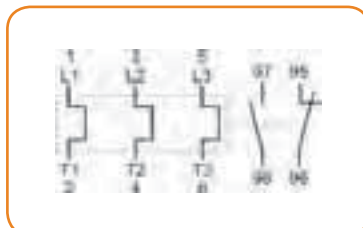
Схема подключения
