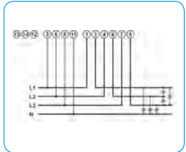
4и – трехфазное, четырехпроводниковое, несимметричная нагрузка
