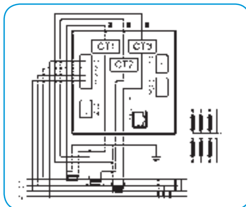
4u – трехфазное, четырехпроводниковое, несимметричная нагрузка
