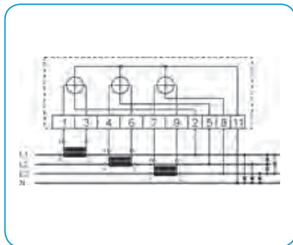
4u – трехфазное, четырёхпроводниковое, несимметричная нагрузка
