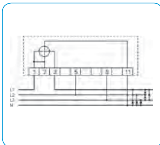
4b – трехфазное, четырехпроводниковое, симметричная нагрузка
