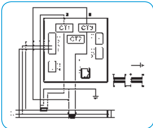
3u – трехфазное, трехпроводниковое, несимметричная нагрузка
