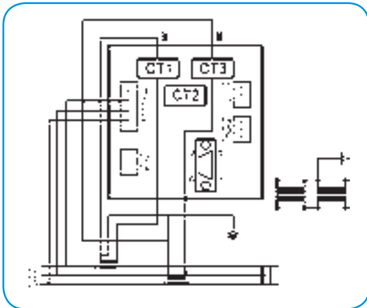
3и – трехфазное, трехпроводниковое, несимметричная нагрузка
